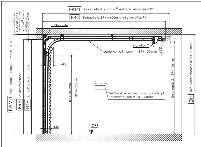
Alle Angaben in mm. Die Dichtung der Sturzblende kann die lichte Durchfahrtshöhe (LDH) um 25 mm verringern.
