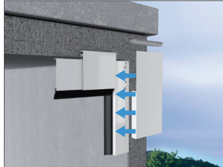
Universal-Blendenlösung, Außenansicht
