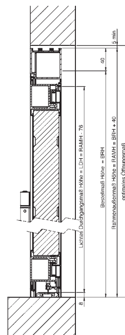
Vertikalschnitt/ Einbau in der Öffnung
