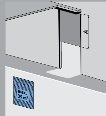
T 500 (B550), Schienensystem mit Vertikalführung
