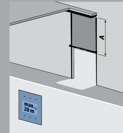
T 500 hF (B550), Schienensystem mit Vertikalführung, mit unten liegender Federwelle + Stahl- Trageprofil
