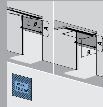
T 500 DS (B350 dock), Schienensystem mit Vertikalführung, mit unten liegender Federwelle
