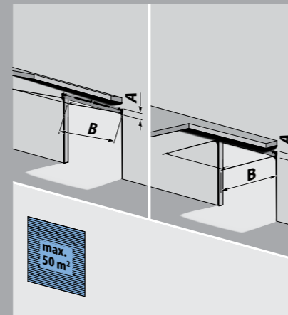
T 450 (B45), Schienensystem mit Normalführung (Standard)
