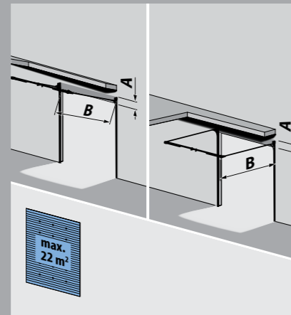
T 340 (B34), Schienensystem mit Normalführung, Federaggregat hinten + Stahl-Trageprofil
