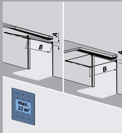
T 240 (B24), Niedrigsturz- Schienensystem, innen- liegende Drahtseile + Stahl-Trageprofil
