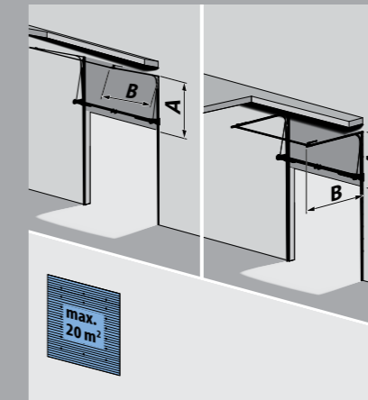
T 400 hF (B350), Schienensystem mit Höherführung, mit unten liegender Federwelle + Stahl- Trageprofil
