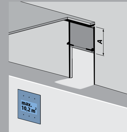
T 500 DS (B550 dock), Schienensystem mit Vertikalführung, mit unten liegender Federwelle
