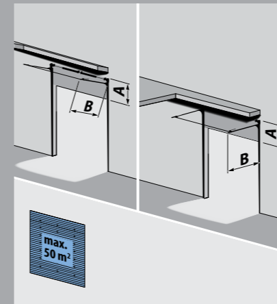
T 400 (B350), Schienensystem mit Höherführung
